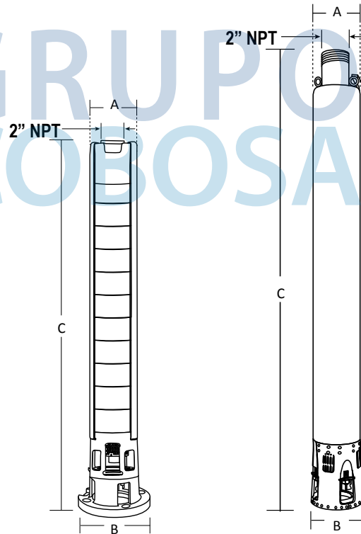
Acoplamiento NEMA 6"
